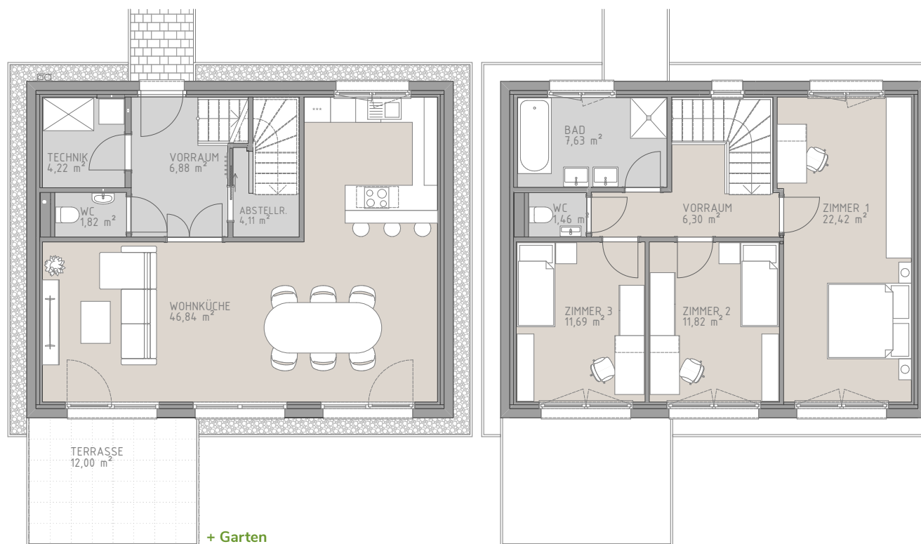
Einfamilienhäuser 4 + 5 WNFL 126,32 m² | Beispiel-Grundriss EFH 4
