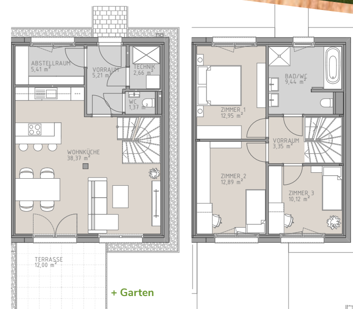
Doppelhaushälften 1 WNFL 102,26 m² | Beispiel-Grundriss 1A
